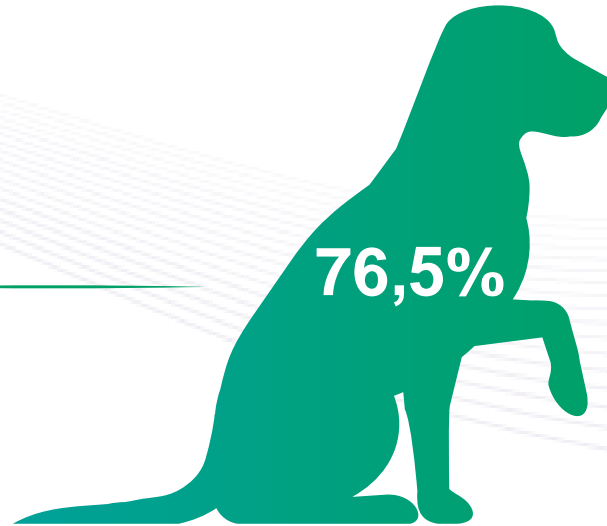
of dog (hair) allergen Can f1
